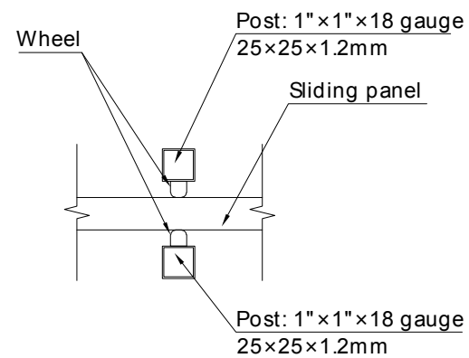
A-A Section
